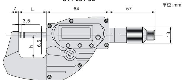
直进式测头
