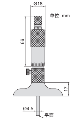
测杆(标配)
